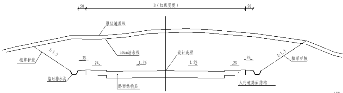
图 2.1-8 一般挖方路基设计图
