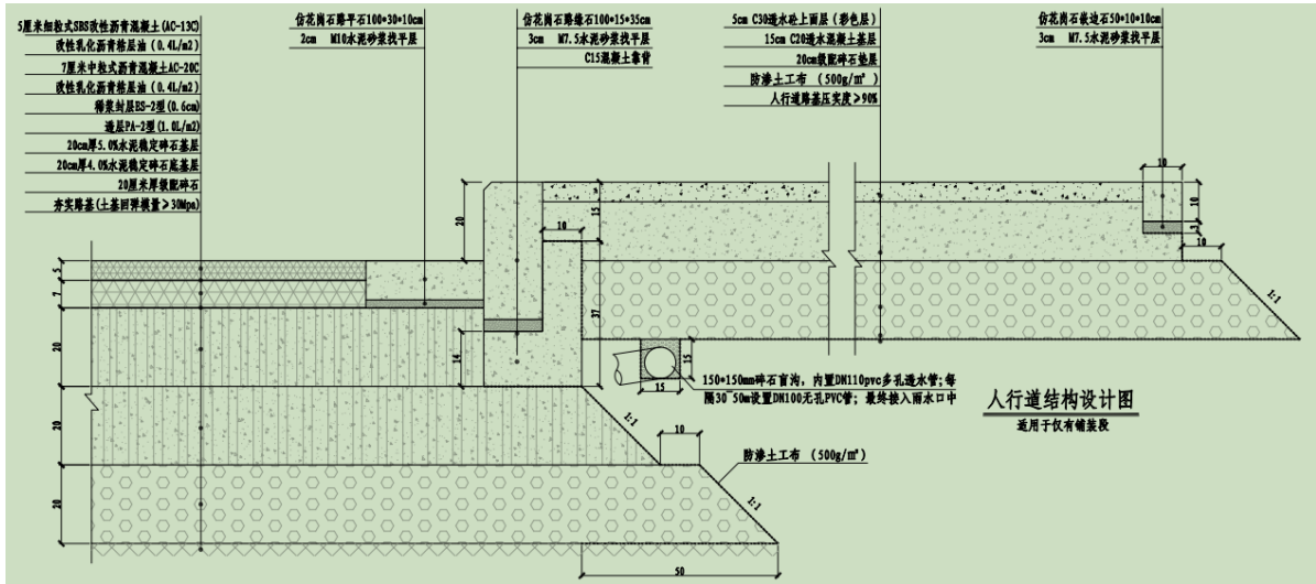
图 2.1-6 路面结构设计图
