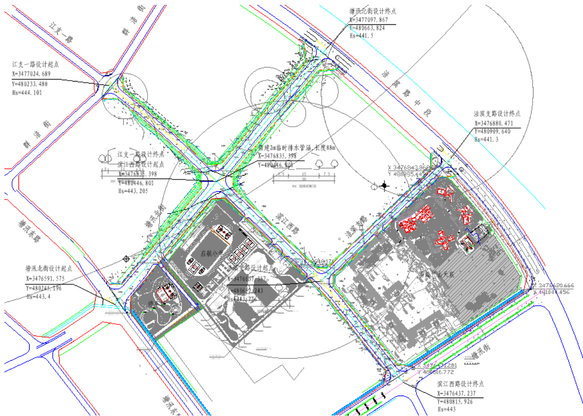
图 2.1-2 道路平面布置图
