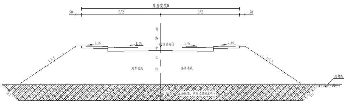
图 2.1-9 特殊路基处理设计图
